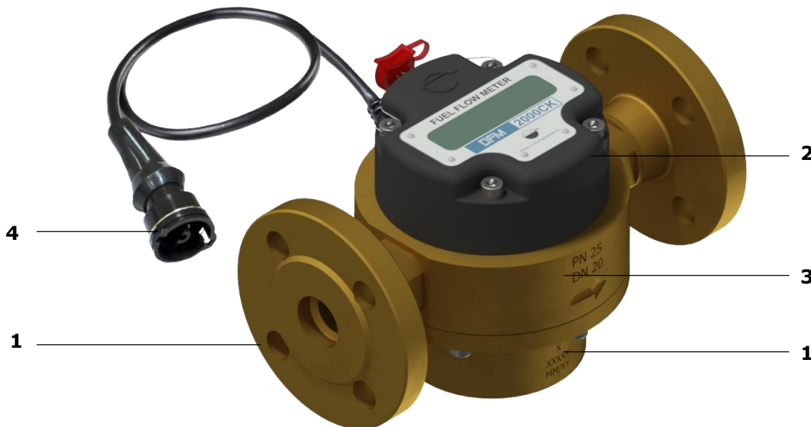
Рисунок 8 — Составные части DFM Marine
