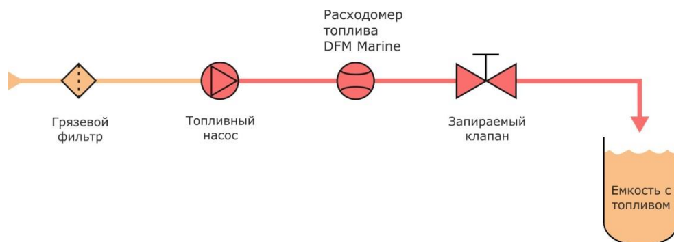
Рисунок 24 — Схема для дозирования порций топлива
