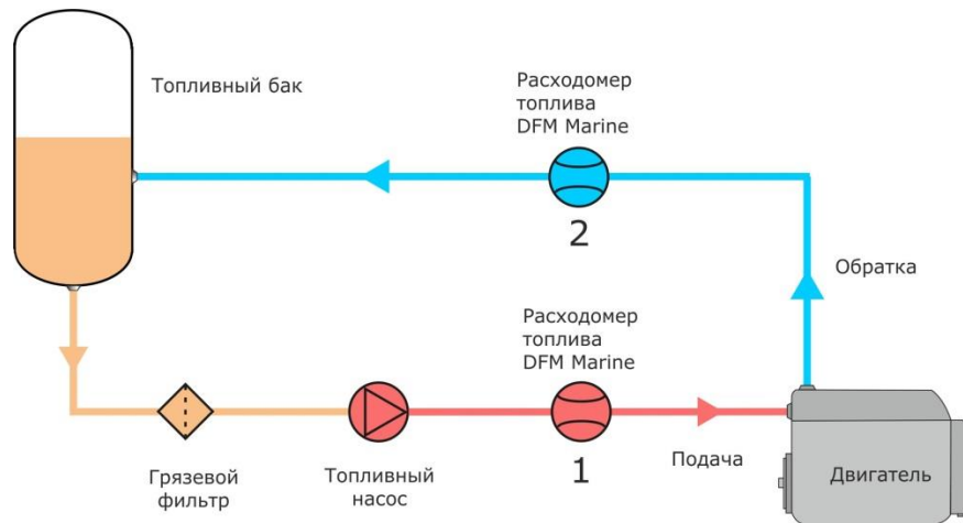
Рисунок 22 — Пример схемы установки DFM Marine «Дифференциальная»
