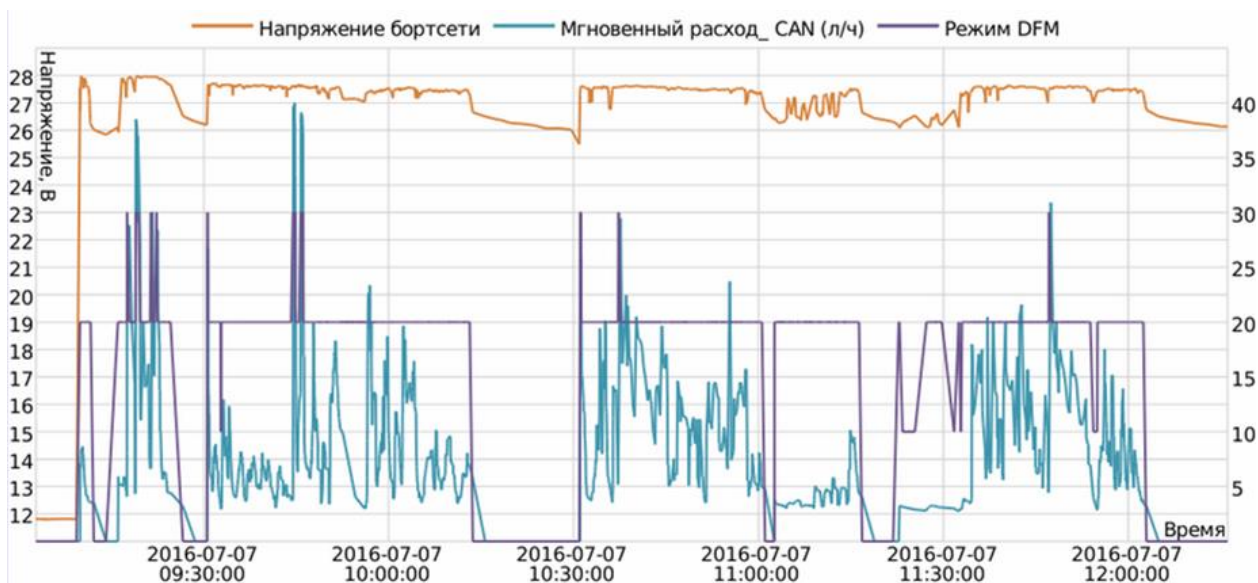
Рисунок 4 — Пример Аналитического отчета, сформированного ORF 4 на основании данных расходомеров топлива DFM Marine CAN
