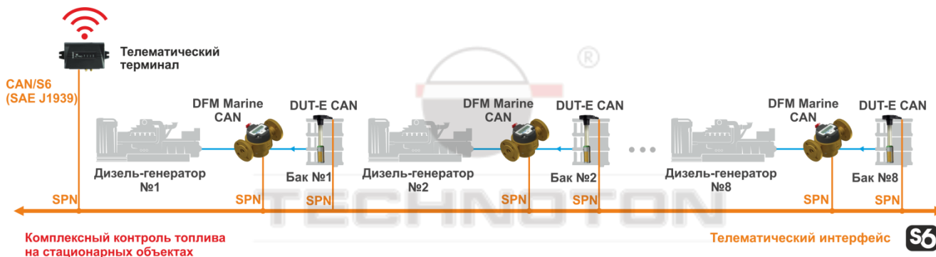
в) пример использования DFM Marine в составе Телематического интерфейса S6 *
